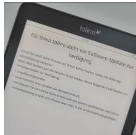
tolino_SW_12.2.jpg:
